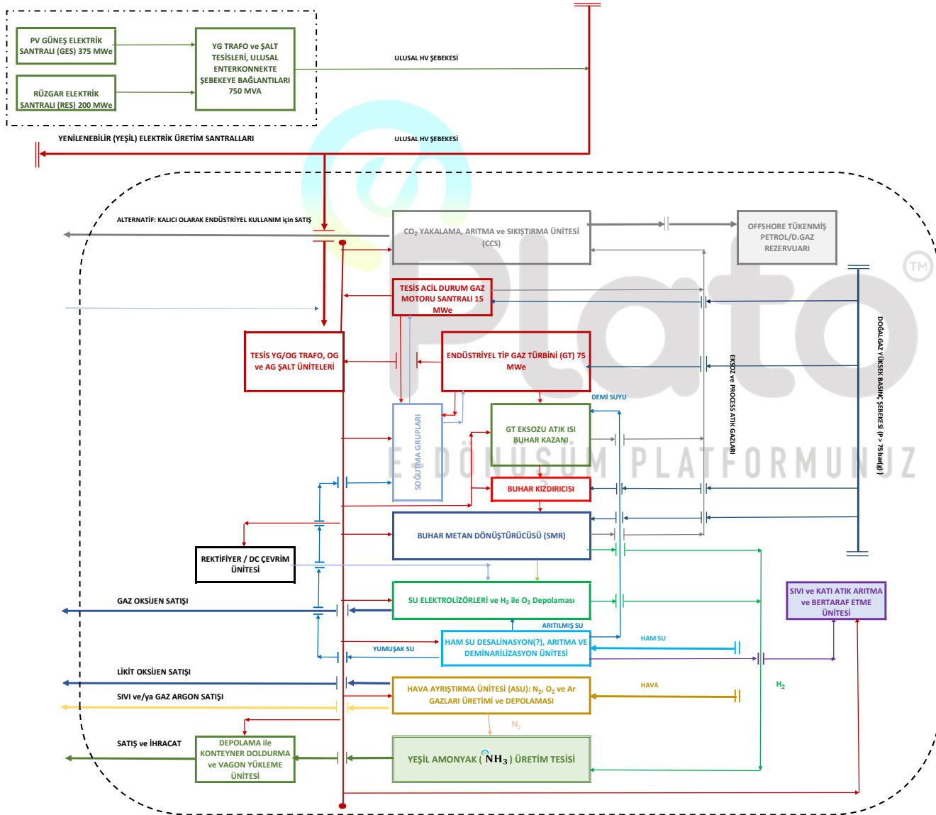
ENTEĞRE 425.000 TON/YIL YEŞİL AMONYAK ( \text{NH}_3 ) ÜRETİM KOMPLEKSİ ANA AKIŞ DİYAGRAMI
